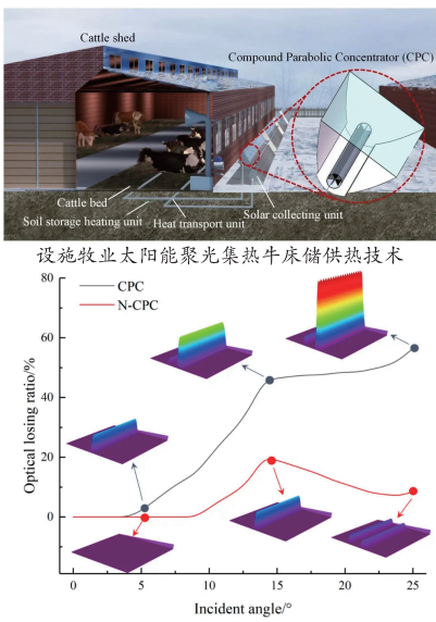
设施农业太阳能聚光电热耦合供能装置性能对比
